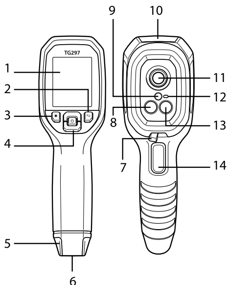
Figure 4.1 Description de la caméra thermique infrarouge (TG297 illustrée)
