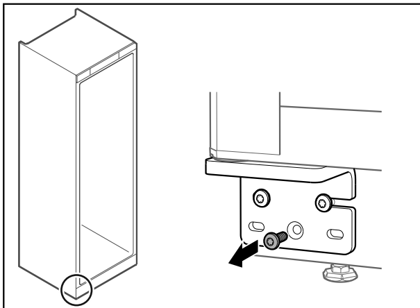
Fig. 61 Congélateur
