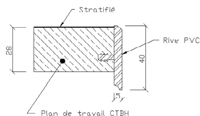
Détail en coupe du plateau
