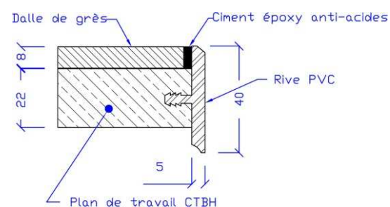
Détail en coupe du plateau
