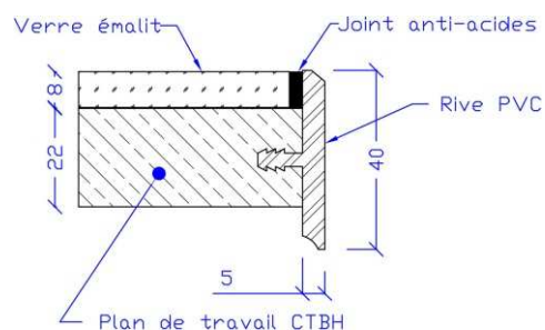
Détail en coupe du plateau
