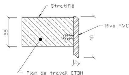
Détail en coupe du plateau
