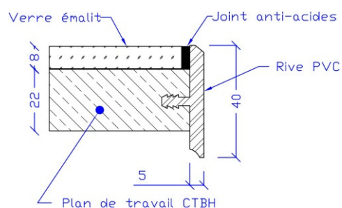
Détail en coupe du plateau
