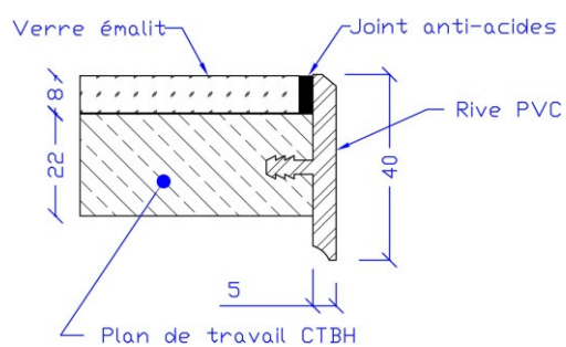
Détail en coupe du plateau
