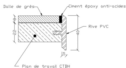
Détail en coupe du plateau
