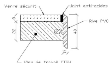
Détail en coupe du plateau
