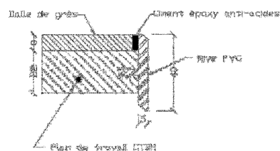
Détail en coupe du plateau
