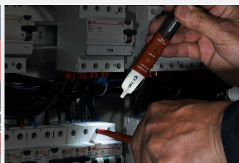
Éclairage de travail intégré (NCV-1030-EUR VOLTfix, NCV-1040-EUR MAGNO-VOLTfix)
