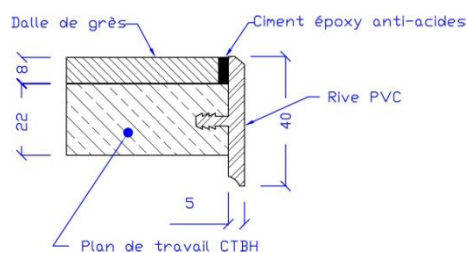
Détail en coupe du plateau
