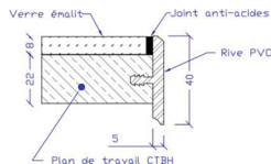
Détail en coupe du plateau
