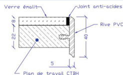
Détail en coupe du plateau
