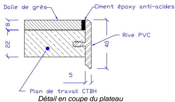
Détail en coupe du plateau
